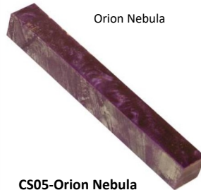
CS05-Orion Nebula
